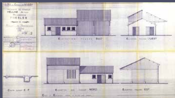
Plan du permis de construire de la ferme de M. Armand Heuline, architecte Félix Ouvré, déposé le 6 mai 1954. Archives départementales du Calvados, 1558W418
